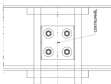
UTSÄTTNING ( 1:5 )
