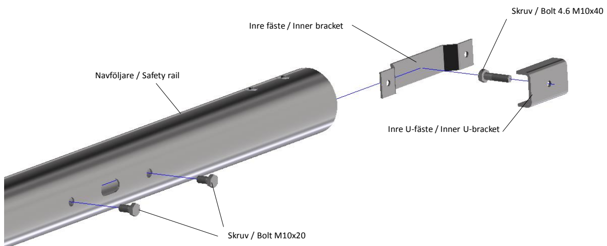
Navföljare med M10 skruv / Safety rail with M10 bolt
